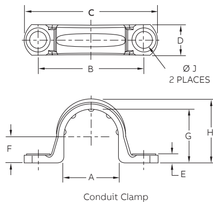
Conduit Clamp
