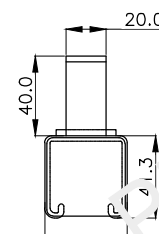
SOPORTE TIPO P3261 - VISTA TRANSVERSAL
