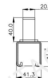
SOPORTE TIPO P3264 - VISTA TRANSVERSAL
