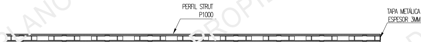
SOPORTE TIPO P3261 - VISTA DE PLANTA
