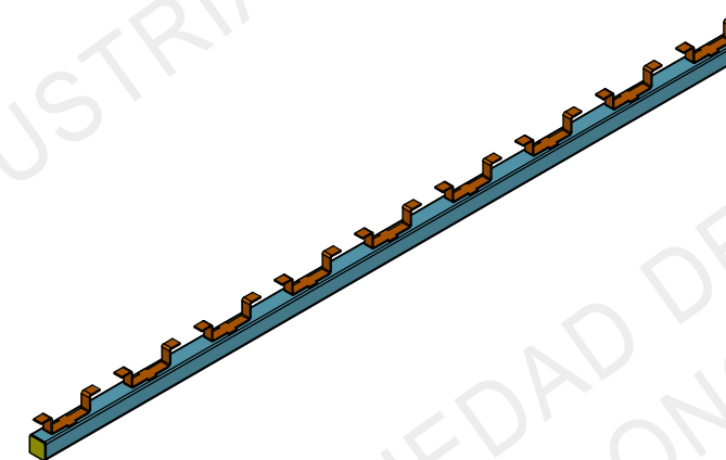
SOPORTE TIPO P3261 - VISTA ISOMETRICA
