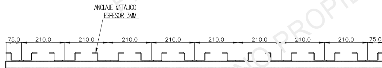
SOPORTE TIPO P3261 - VISTA LATERAL
