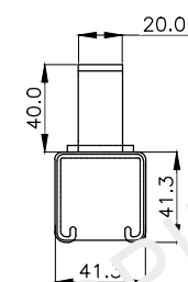
SOPORTE TIPO P3260 - VISTA TRANSVERSAL ESC: S/E
