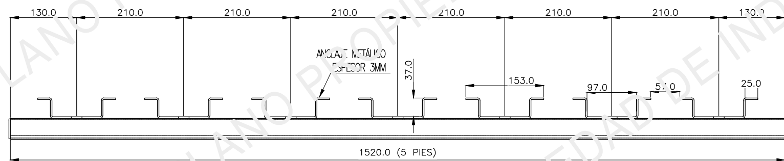
SOPORTE TIPO P3260 - VISTA LATERAL ESC: S/E
